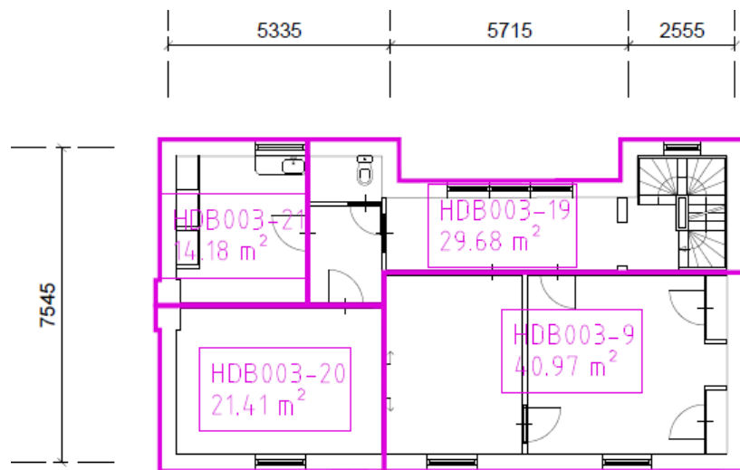
1 e verdieping
